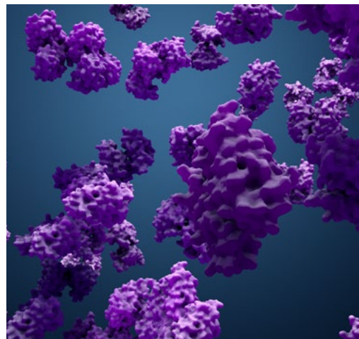
Denaturazione delle proteine e inattivazione delle RNasi
